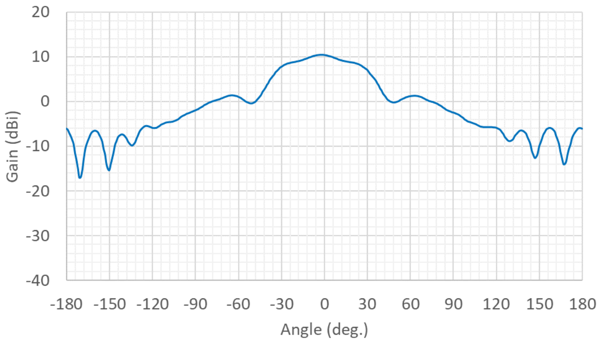
5GHz (E-Plane)
