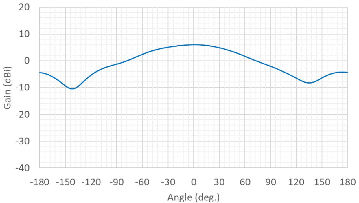
1GHz (E-Plane)
