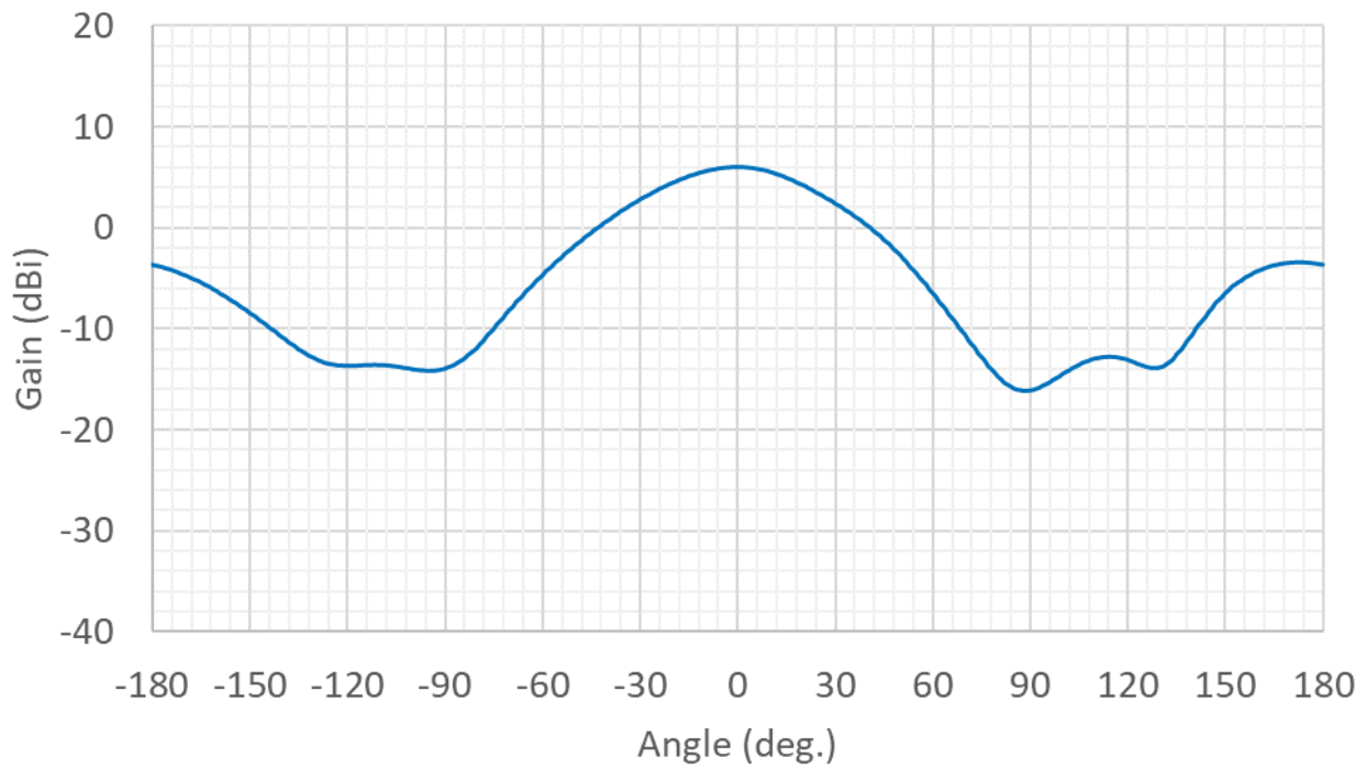
1GHz (H-Plane)
